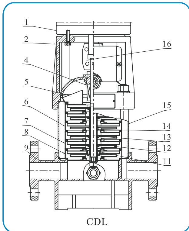
截面图 CDL,CDLF 1,2,3,4,5
