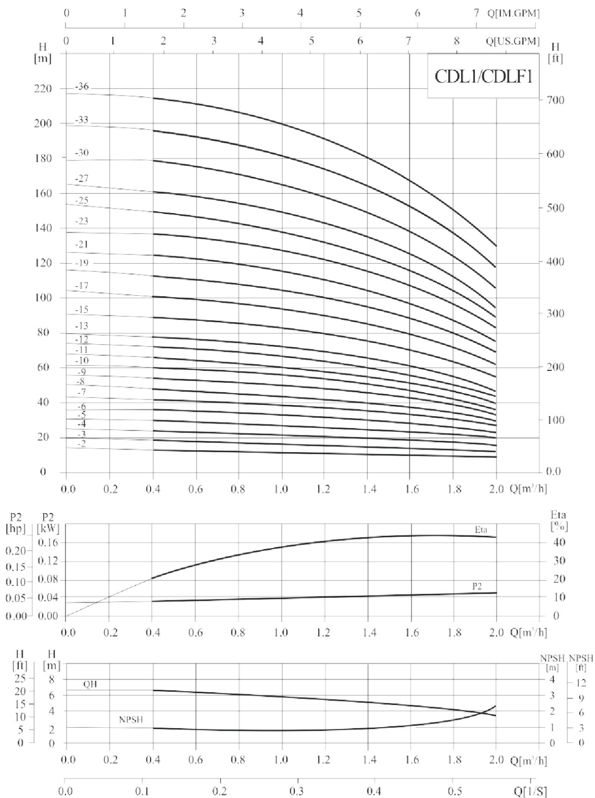
性能曲线
