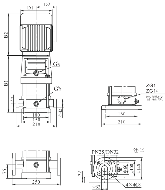
安装图
