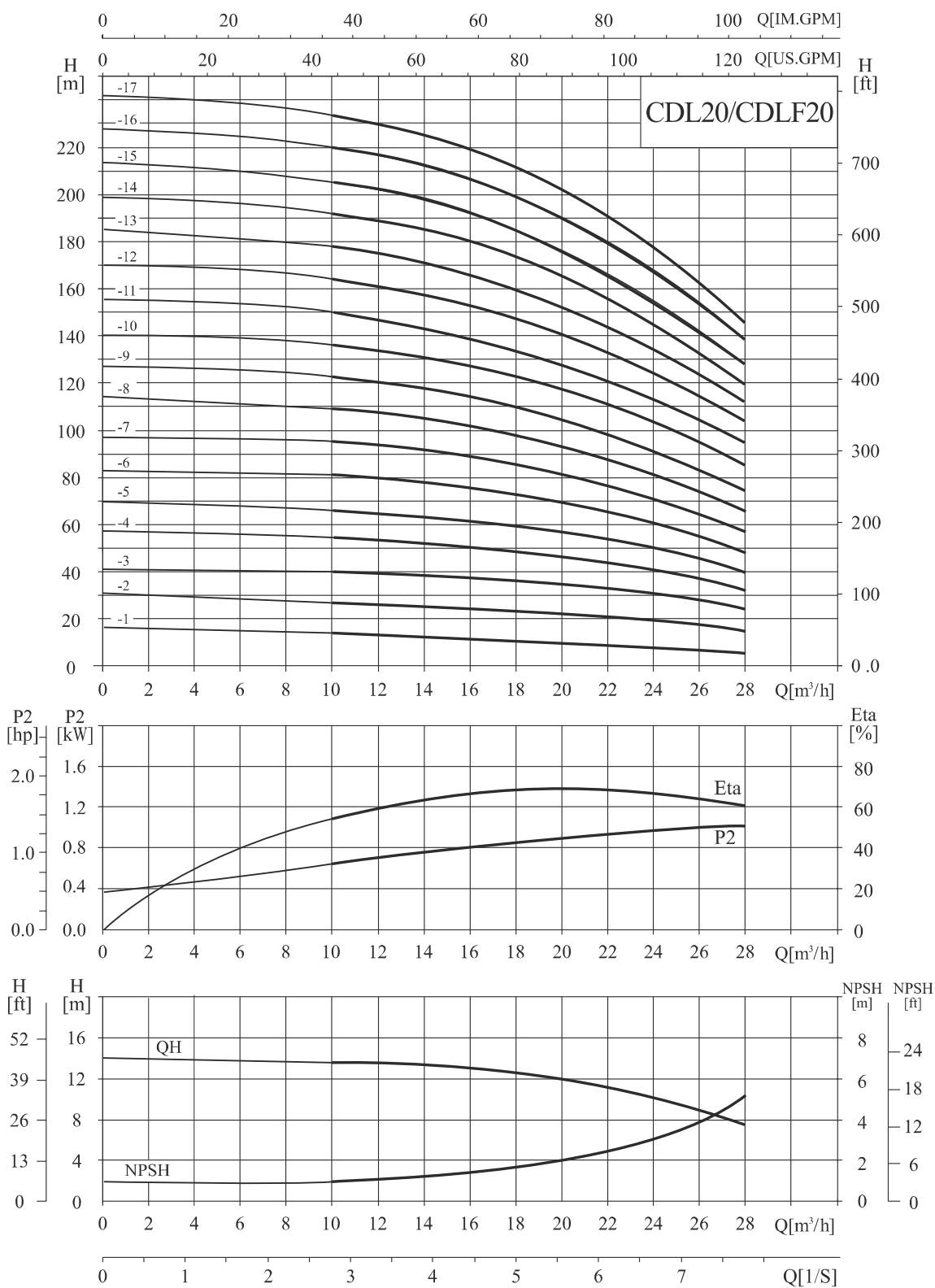
性能曲线
