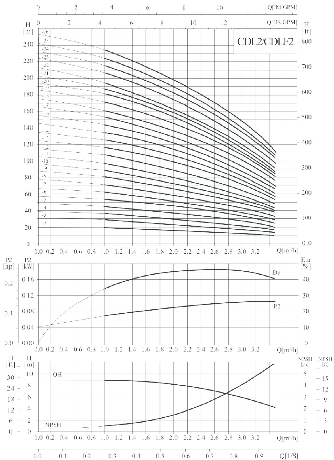
性能曲线
