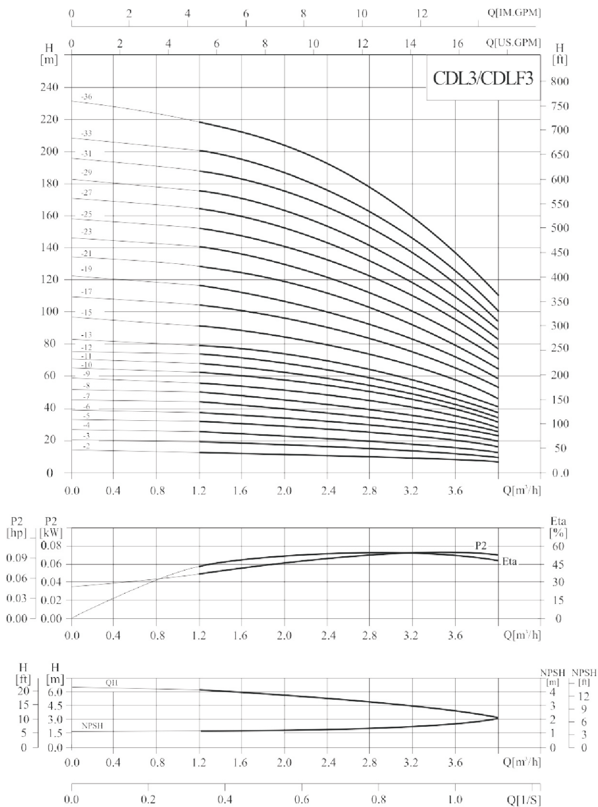
性能曲线
