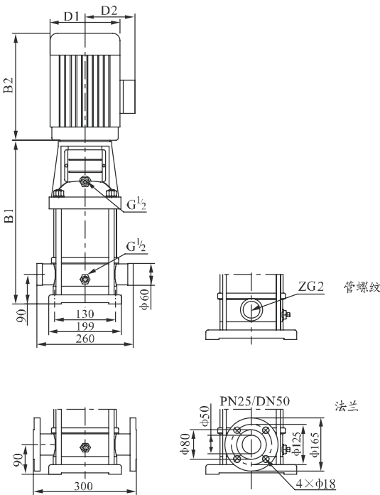
安装图
