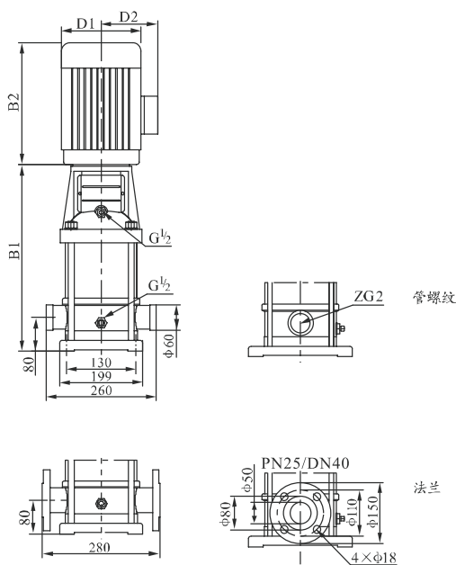
安装图
