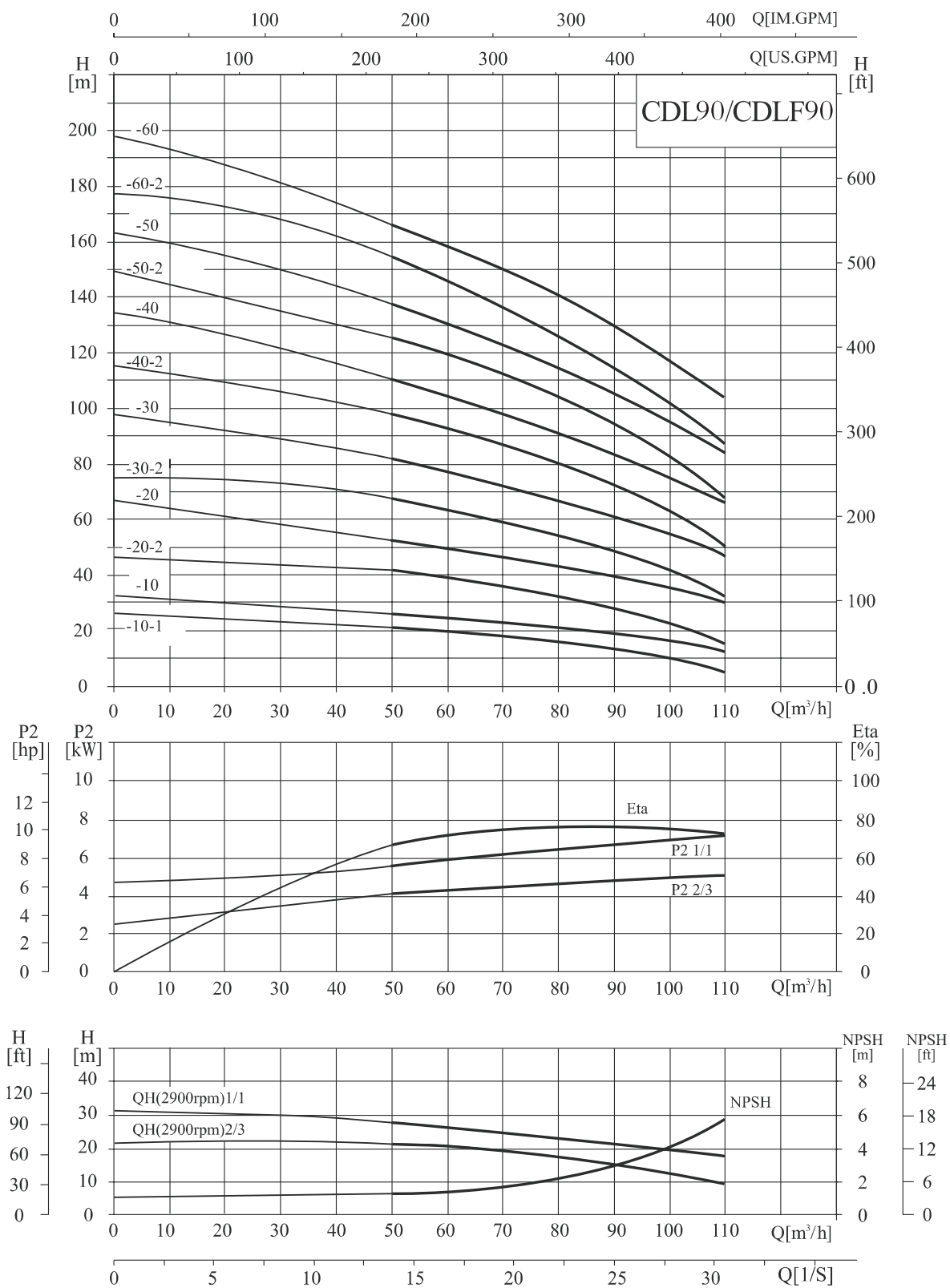
性能曲线
