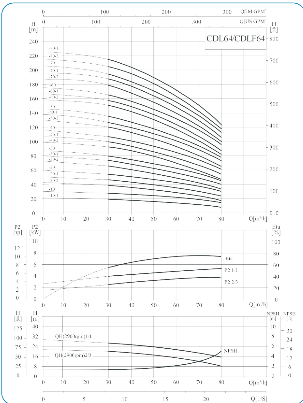
性能曲线
