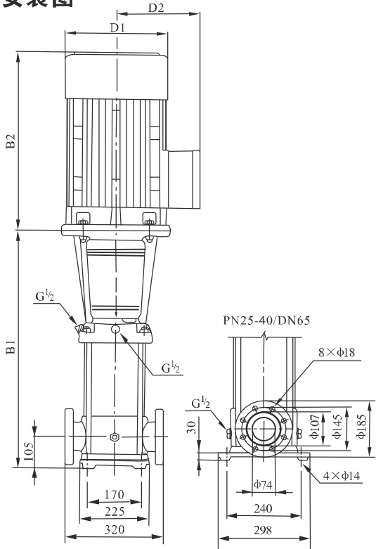
安装图
