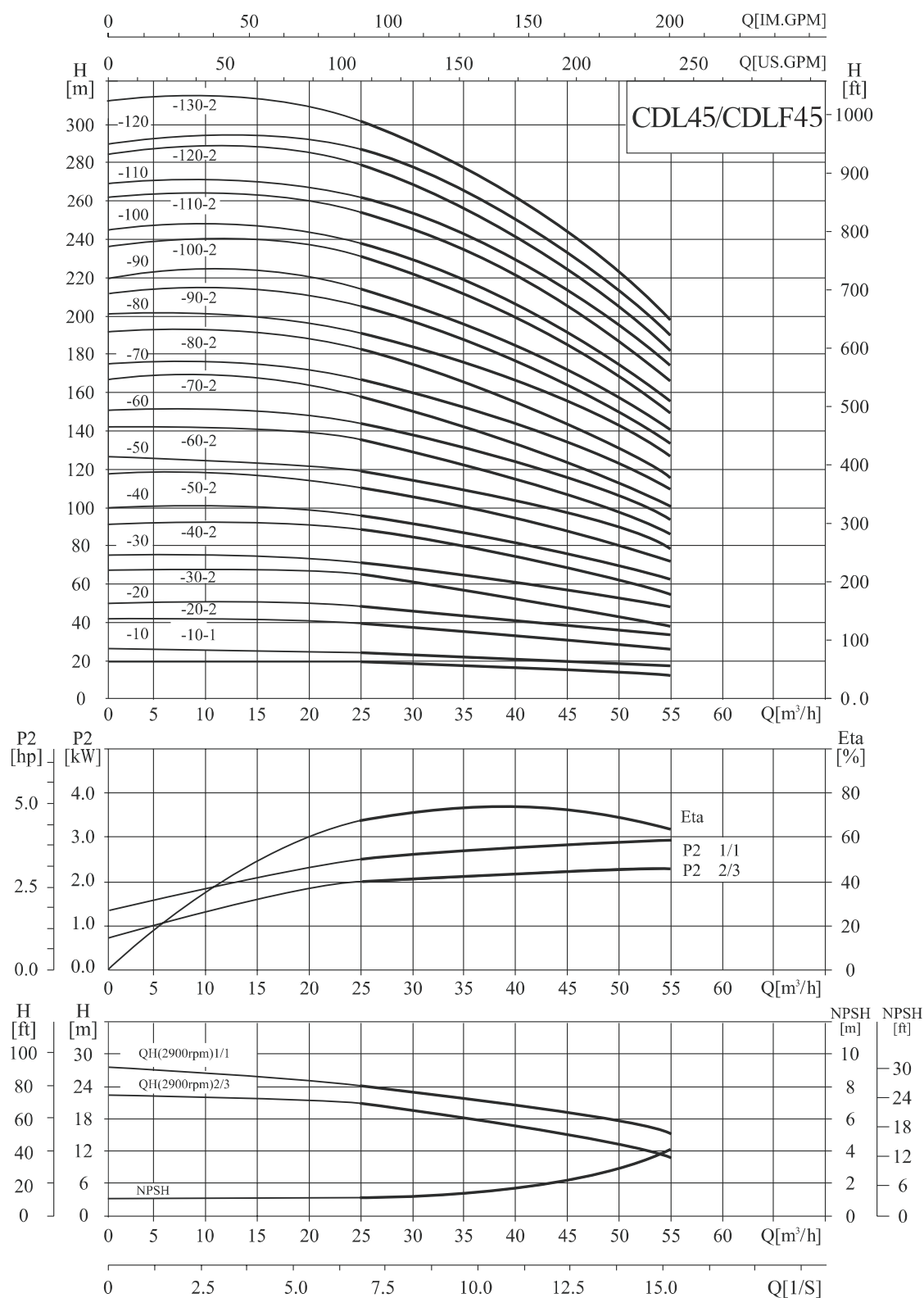
性能曲线
