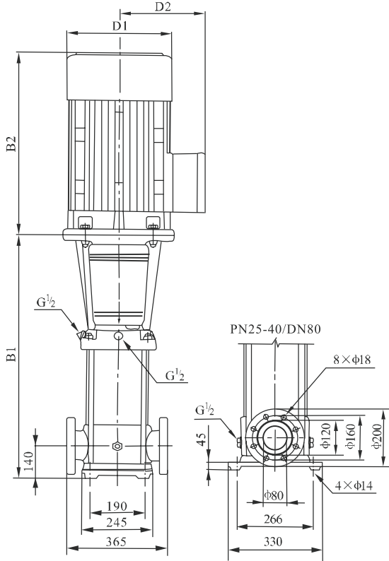
安装图
