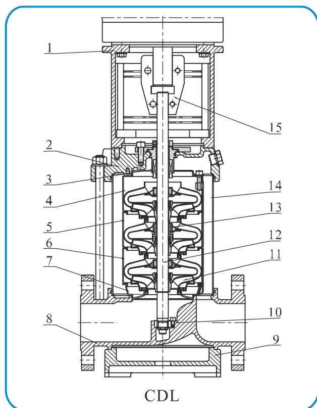
截面图 CDL,CDLF32,45,64,90
