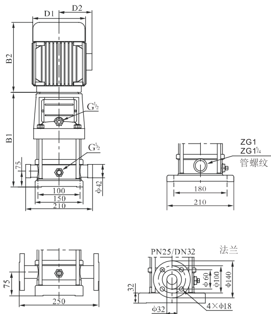
安装图
