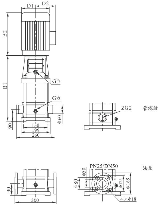
安装图
