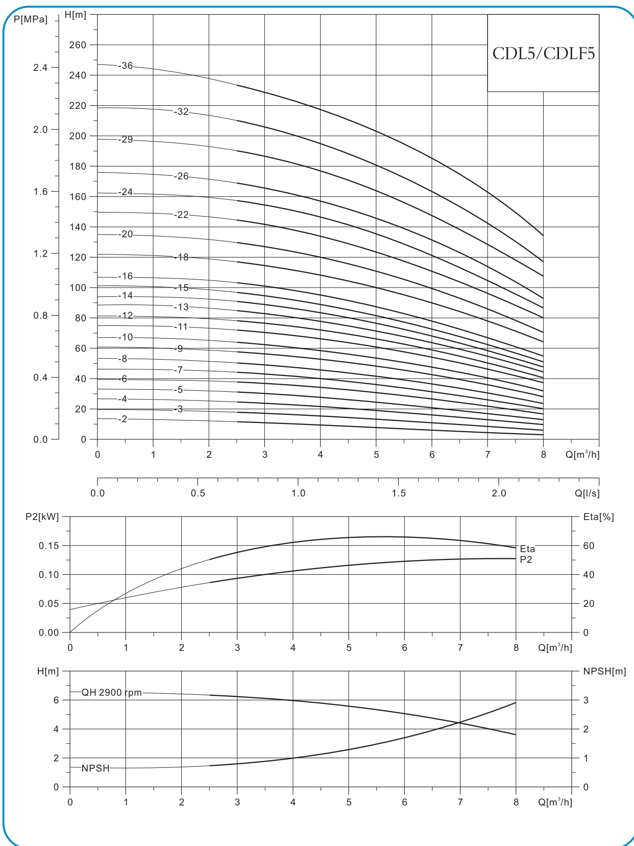
性能曲线
