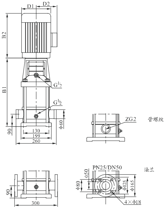
安装图
