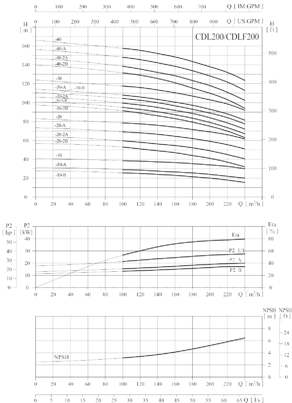
性能曲线
