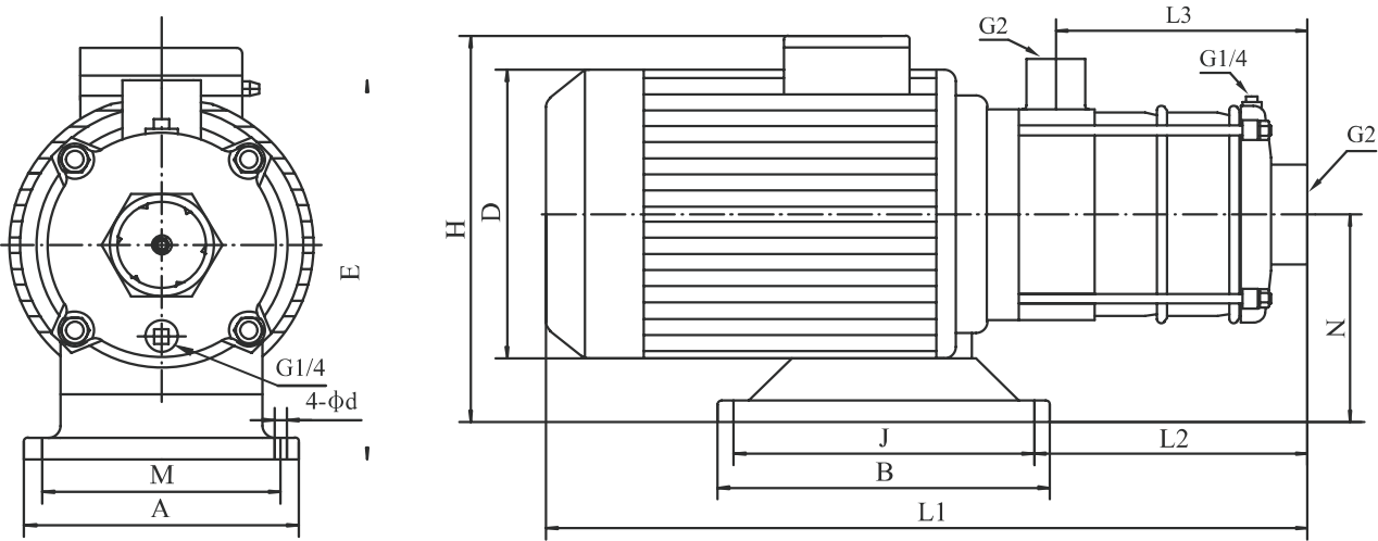
尺寸和重量
