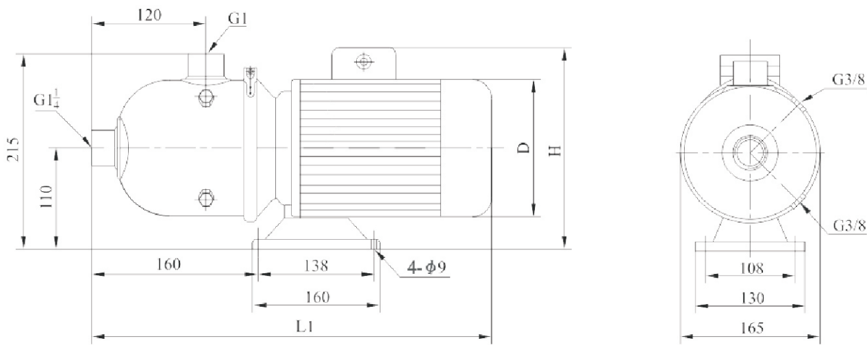
安装图
