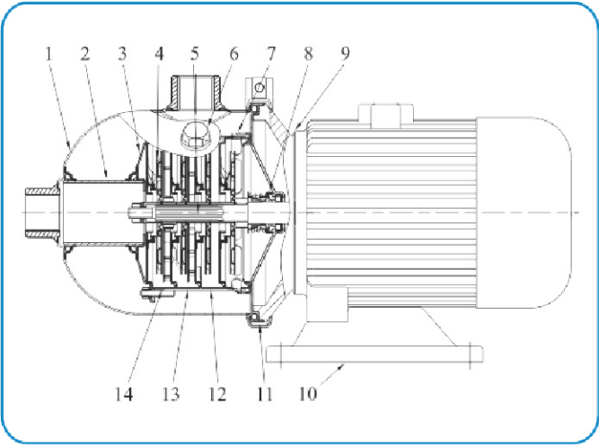
截面图 CHL 2,4
