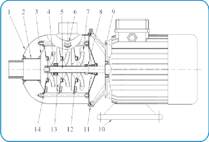
截面图 CHL8,12,16,20
