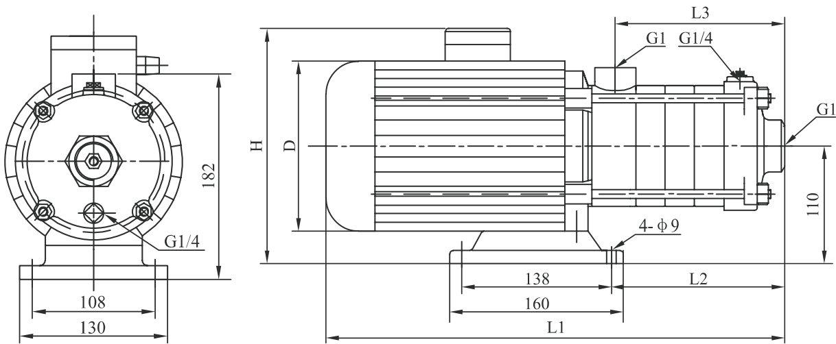
尺寸和重量
