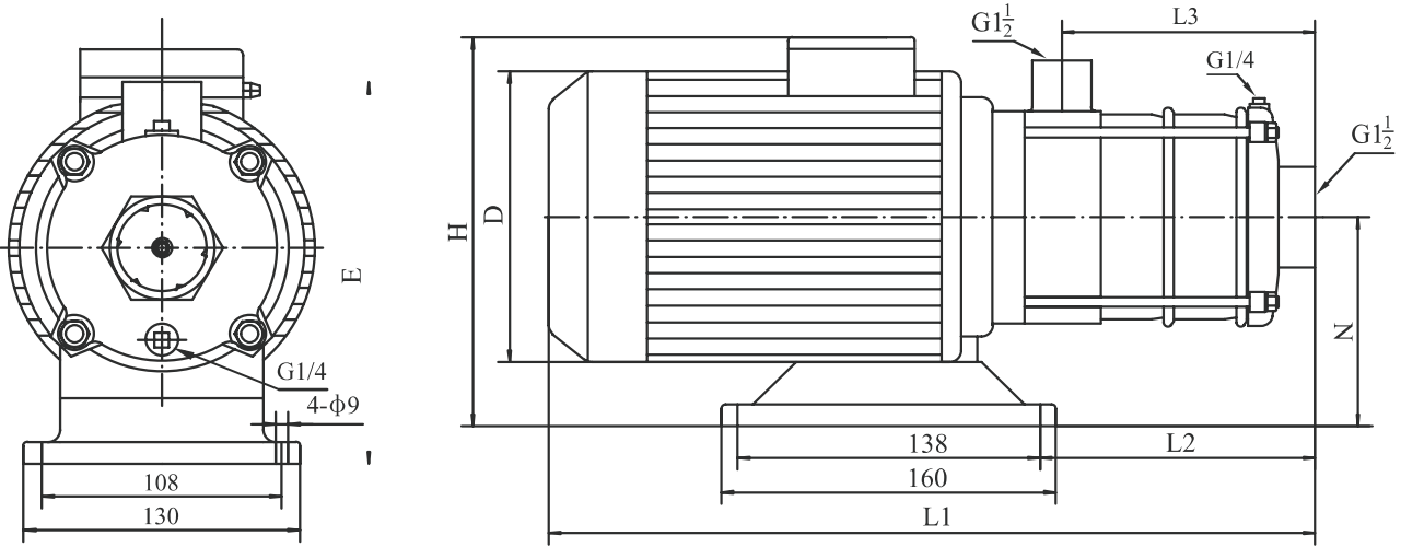
尺寸和重量
