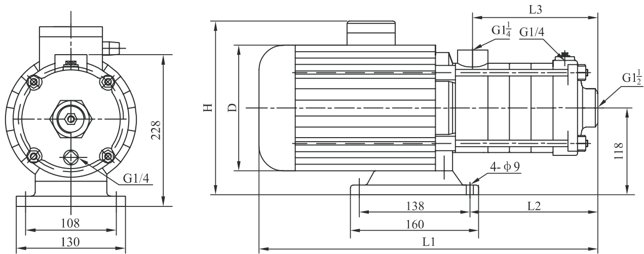
尺寸和重量
